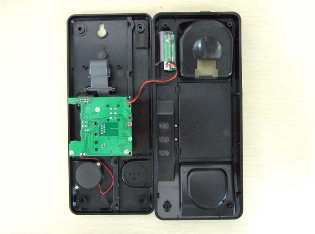
PCB1
