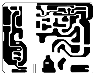
Bottom Layer
