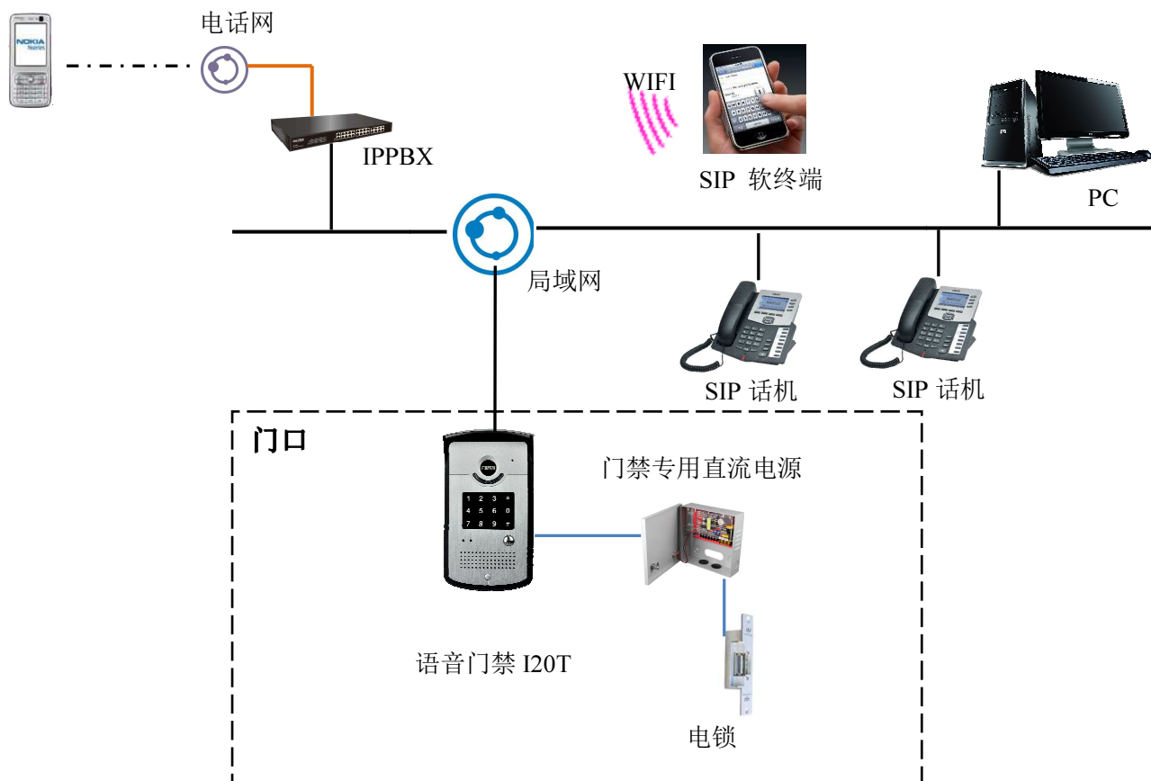
系统组成框图
